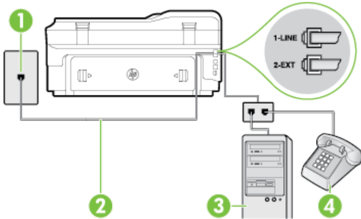
打印机的后视图
